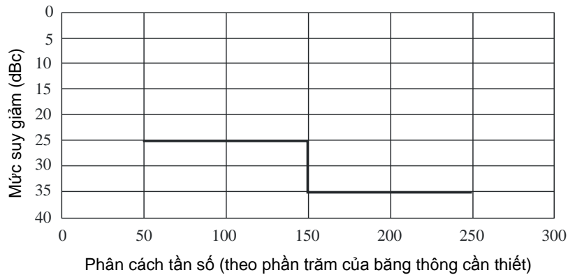
Hình D.16 - Mặt nạ phổ phát xạ ngoài băng cho nghiệp vụ di động hàng không và hàng hải
