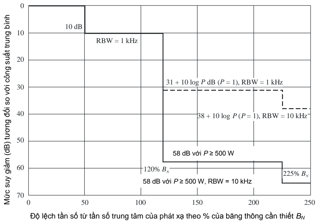
Hình D.10 - Các đòi hỏi trong dải tần trên 30 MHz trong trường hợp băng tiêu chuẩn hoặc băng hẹp của khuyến nghị ITU-R SM.1539
