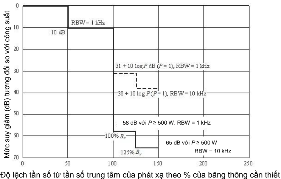
Hình D.11 - Các đòi hỏi trong dải tần trên 30 MHz trong trường hợp băng rộng của khuyến nghị ITU-R SM.1539
