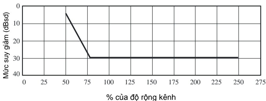
Hình D.12 - Mặt nạ phổ phát xạ ngoài băng cho hệ thống di động mặt đất với độ rộng kênh 12,5 kHz
