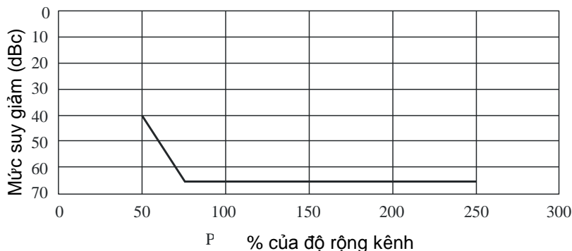
Hình D.13 - Mặt nạ phổ phát xạ ngoài băng cho hệ thống di động mặt đất với độ rộng kênh 5 kHz
