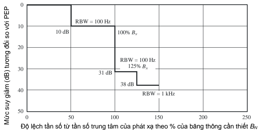
Hình D.9 - Các dải hoạt động trong dải tần dưới 30 MHz trong trường hợp băng rộng của khuyến nghị ITU-R SM.1539
